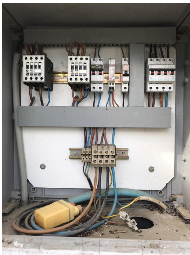
FOTO 1. - Quadro elettrico Q2
