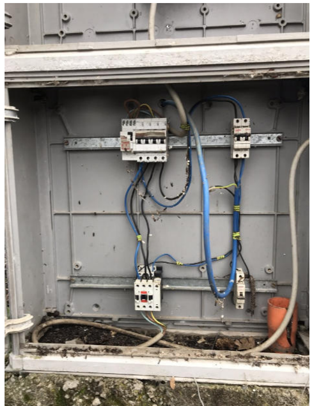
FOTO 2. - Quadro elettrico Q1
