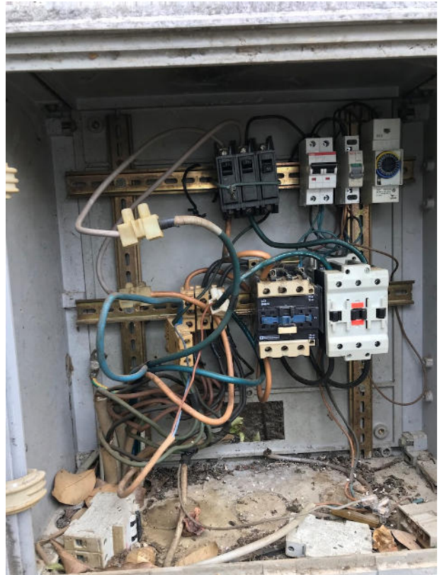
FOTO 2. – Quadro elettrico Q12.
